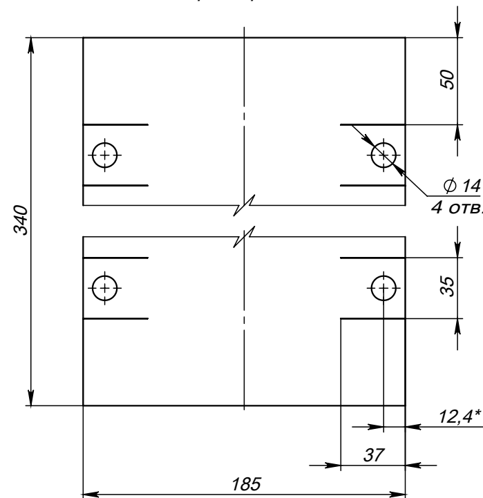
Поз.2 (Ложемент) развертка
