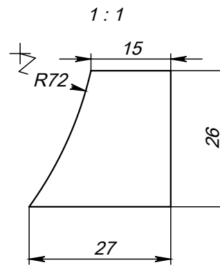
Поз.4 (Ребро ушка)
