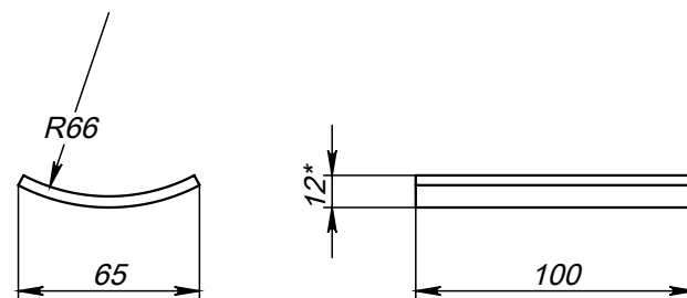
Поз.5 (Упор)
