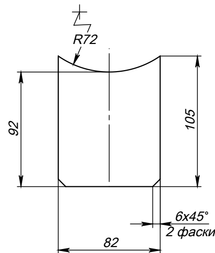
Поз.3 (Ребро)
