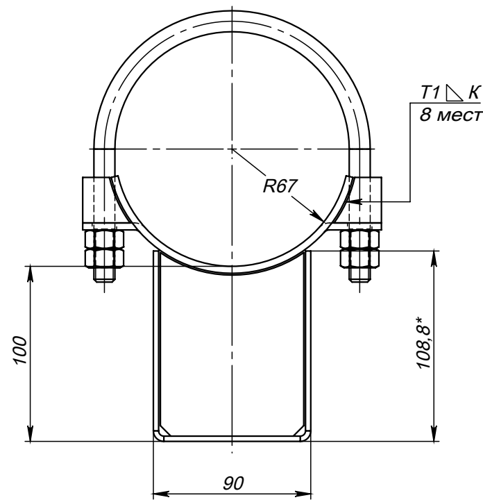
Поз.2 (Ложемент)
