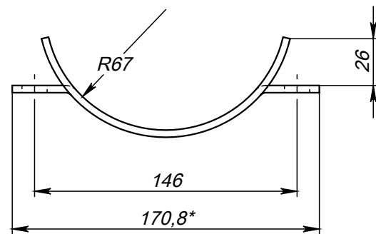
Поз.2 (Ложемент)
